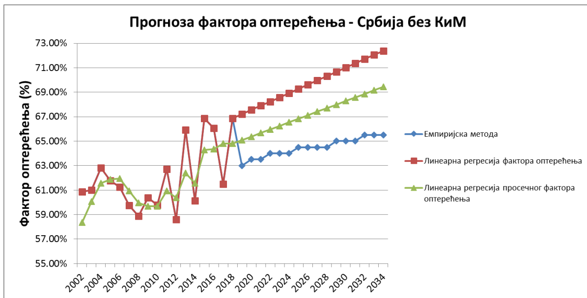
Сл.Д. 4.18: Прогноза фактора оптерећења ЕЕС Републике Србије без конзумног подручја АП КиМ до 2034. године
